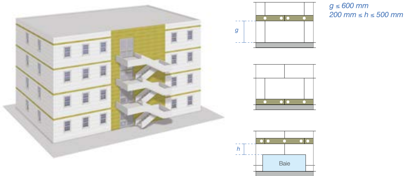
Figure 3// schémas de disposition de la bande filante sur bâtiment (dessin tiré de WAVD)
