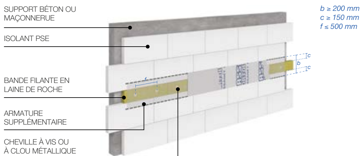
Figure 1// bande filante, dessin tiré d'ETICS-PSE Guide de PRÉCONISATION, avril 2016
