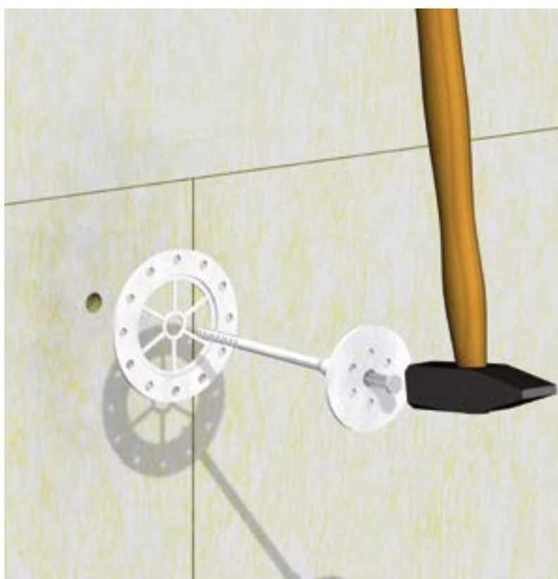
CHEVILLE À PERCUSSION FASSA COMBI FIX, AVEC RONDELLE SUPPLÉMENTAIRE, SUR LAINE DE ROCHE
