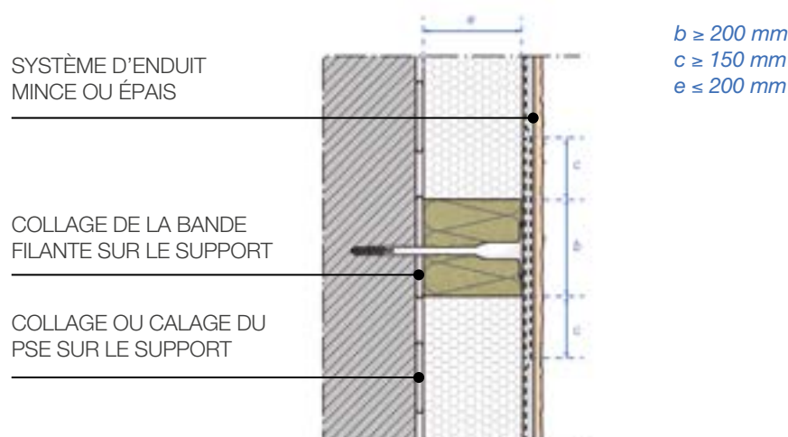
Figure 2// détail de fixation et collage de la bande filante, tiré d'ETICS-PSE Guide de PRÉCONISATION, avril 2016
