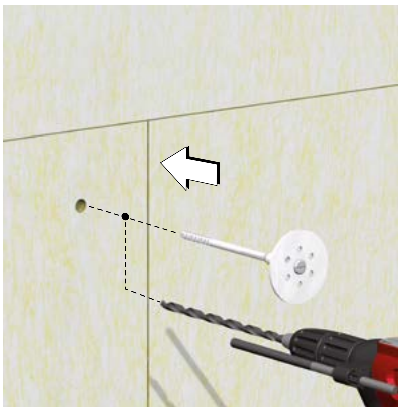
CHEVILLE À PERCUSSION FASSA COMBI FIX, AVEC RONDELLE SUPPLÉMENTAIRE, SUR LAINE DE ROCHE
